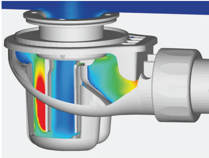
← Virtueller Strömungstest eines extraflachen Siphons für Duschabläufe.
