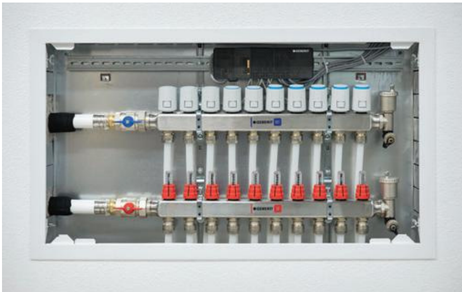
↑ Steuerschrank für das Heizsystem eines Mehrfamilienhauses. In der Mitte oben befindet sich die zentrale Reglereinheit.
